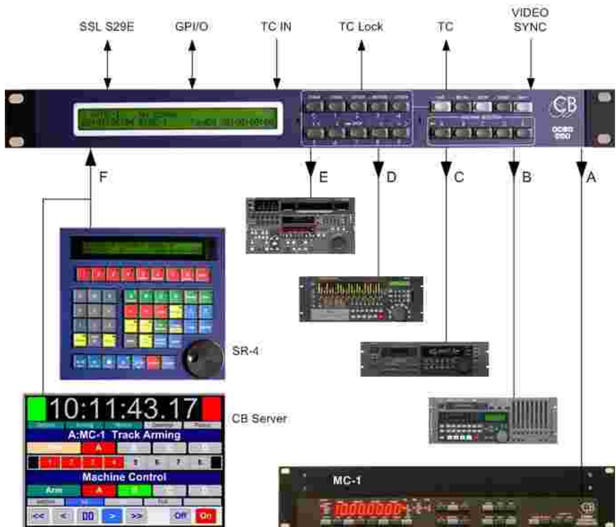
Figure 3: RM-6 exemple de système
